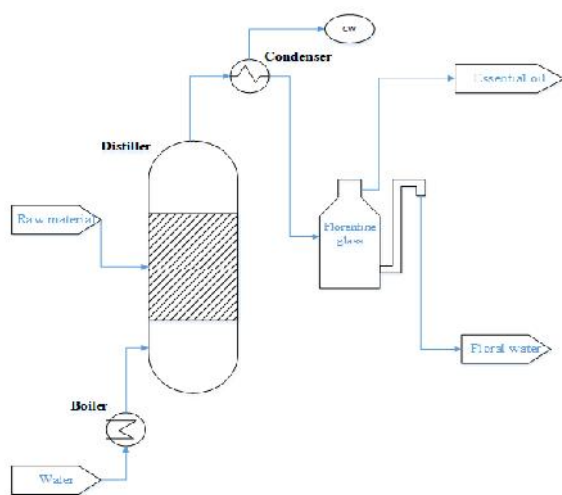
Fig. 1. Esquema del equipo de extracción, adaptado de [15]
